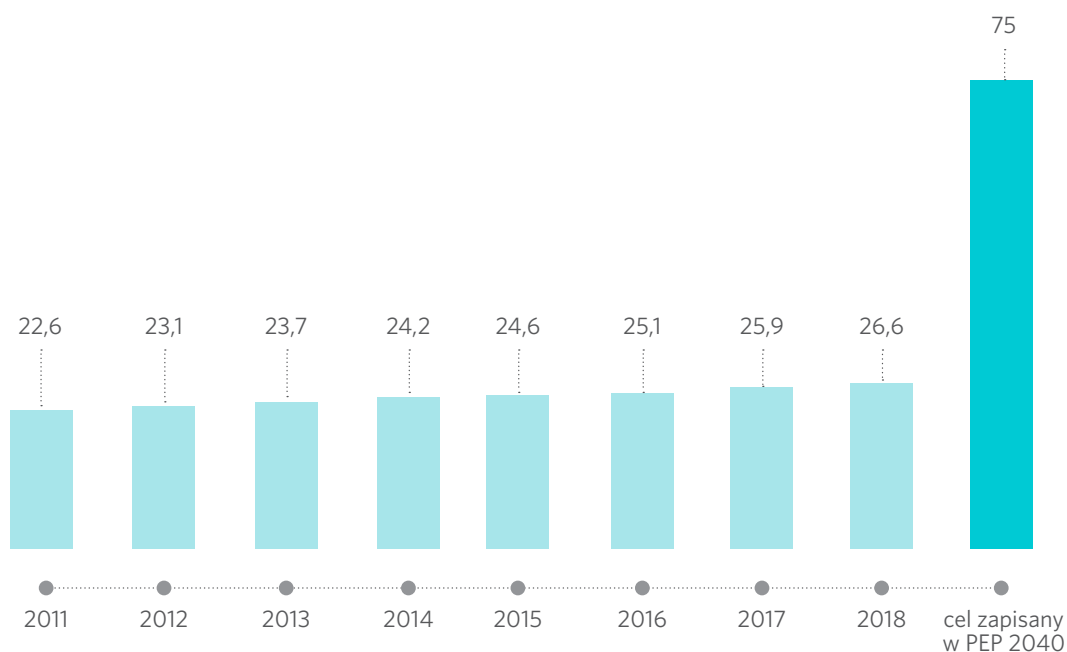
UDZIAŁ LINII KABLOWYCH W LINIACH ŚREDNICH NAPIĘĆ NAJWIĘKSZYCH OSD W POLSCE (W PROC.)
